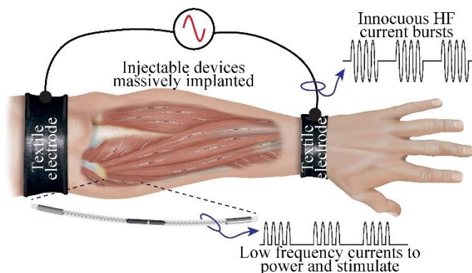
Abb. 2 Der Grundaufbau des intelligenten drahtlosen Netzwerks aus Sensoren und Aktoren. Es besteht aus injizierten Elektroden, externen Textilelektroden und Controllern.
