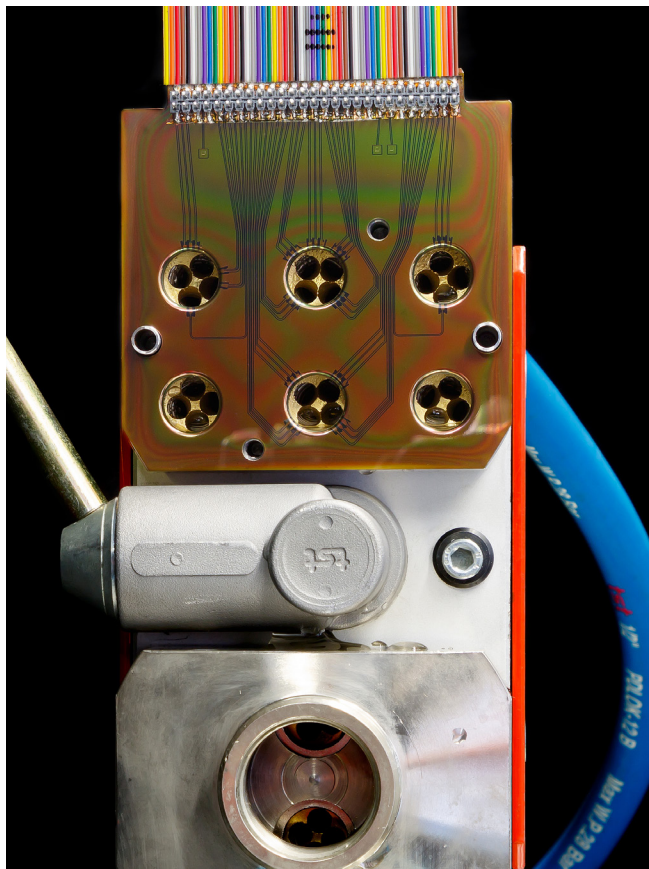
Sensorischer Multikupplungsein- satz zur Überwachung der Tem- perierung. © Fraunhofer IST
