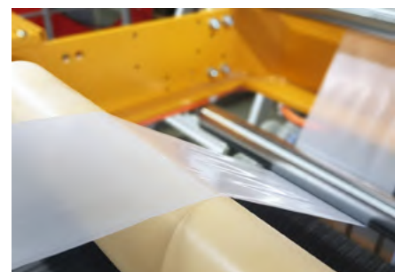
Herstellung einer bio-funktionalisierten Folie im Verarbeitungstechnikum.
